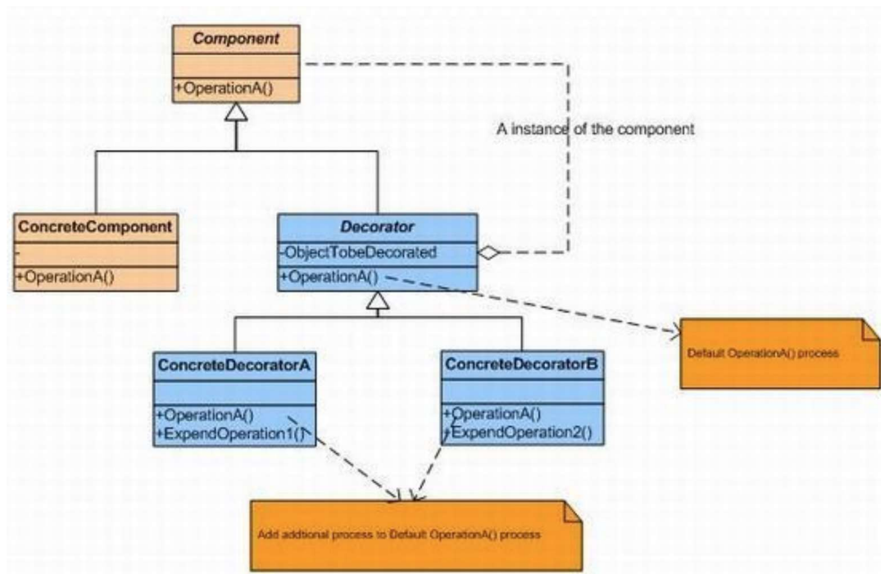
Diagrama UML genérico en un patrón Decorator.
